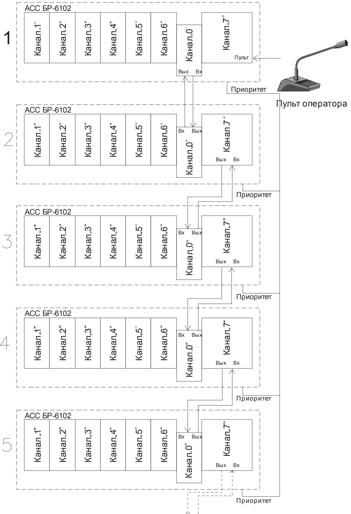
Схема наращивания числа каналов свыше 12
