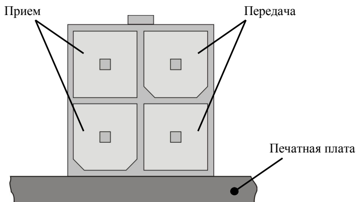
Рисунок 2 - Распайка разъема блока защиты. Вид сверху
