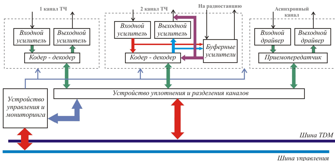
Рисунок 1 - Структурная схема блока выделения каналов V2A1 - R
