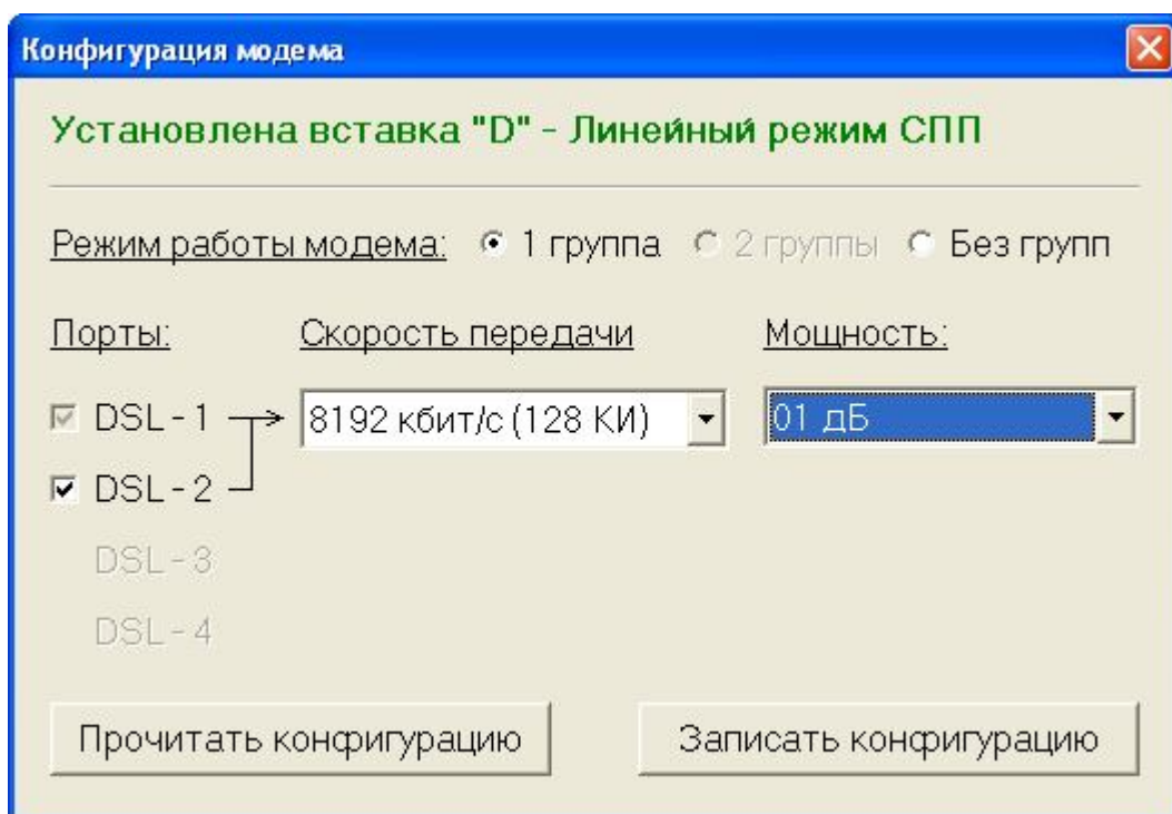
Рисунок 8 Конфигурация модема. Режим “1 группа 2 порта”(ПО “Поток-2”)
