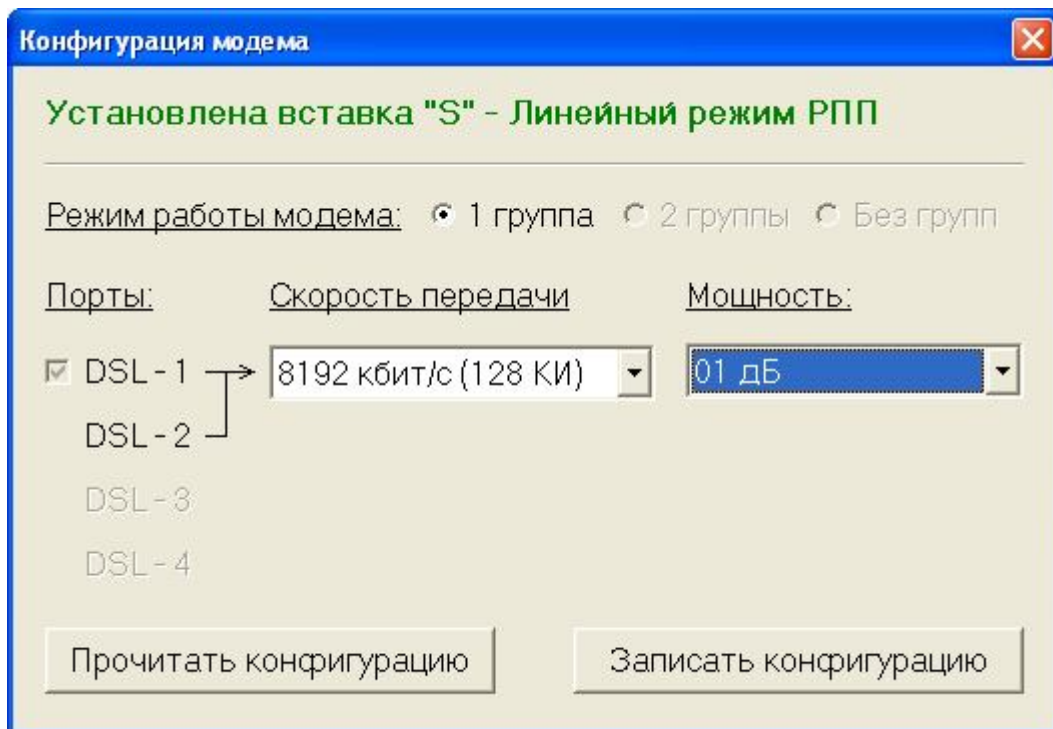
Рисунок 11 Конфигурация модема. Режим "1 группа 1 порт". Линейный режим РПП (ПО "Поток-2")
