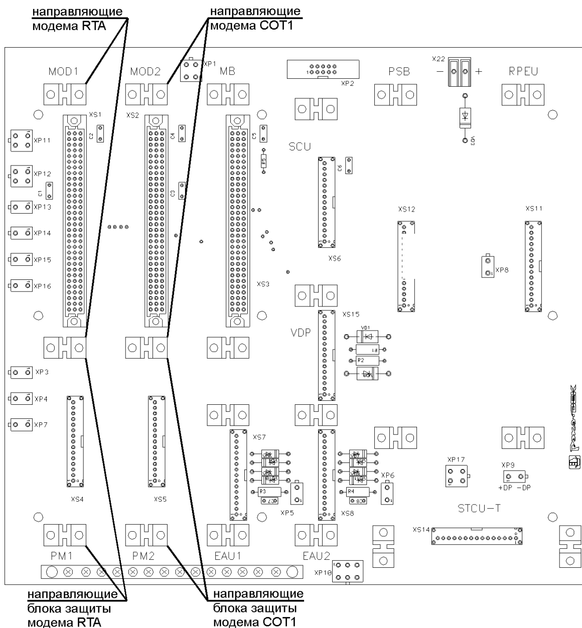
Рисунок 20 Кросс-ТС. Модуль регенерационный REG-ТС
