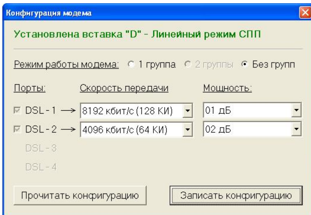
Рисунок 10 Конфигурация модема. Режим “Без групп”. Линейный режим СПП (ПО “Поток-2”)
